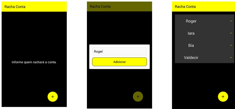
Figura 1.14: Racha Conta
