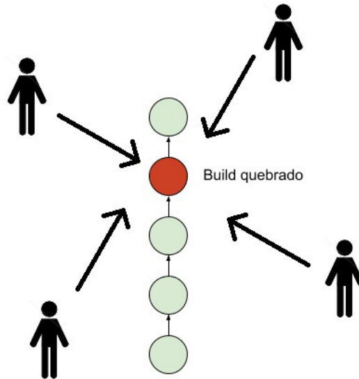
Figura 2.1: Build quebrado
