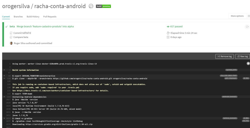
Figura 2.4: Build disparado em software de integração contínua
