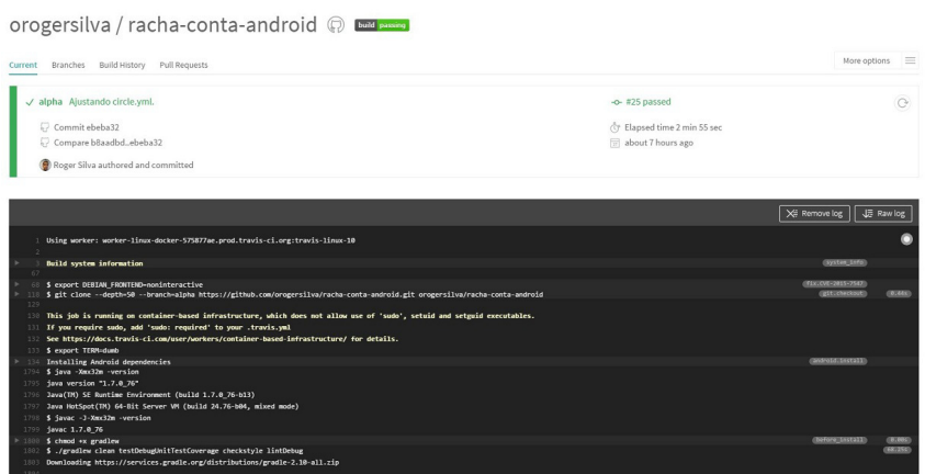
Figura 1.9: Travis CI
