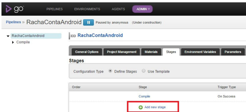
Figura 4.15: Criação de novo stage
