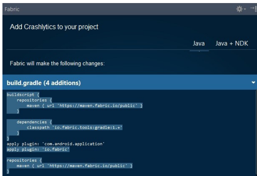
Figura 5.30: Adição de configuração para o Crashlytics
