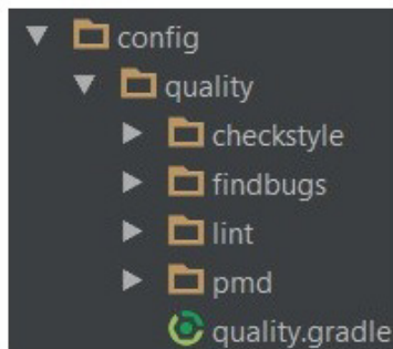
Figura 3.19: Organização de folders para análise estática de código
